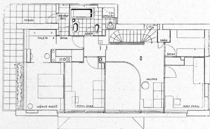
Půdorys patra 1:200.
